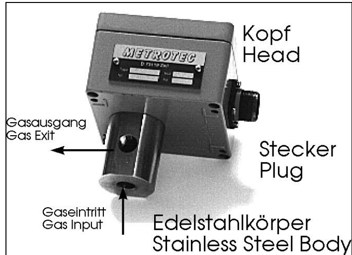
Sensor A15
