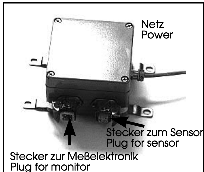
Converter module Z15
