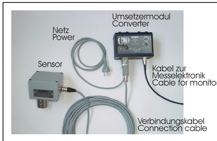
Verschaltung des Sensors A15-N mit dem Umsetzermodule U15
