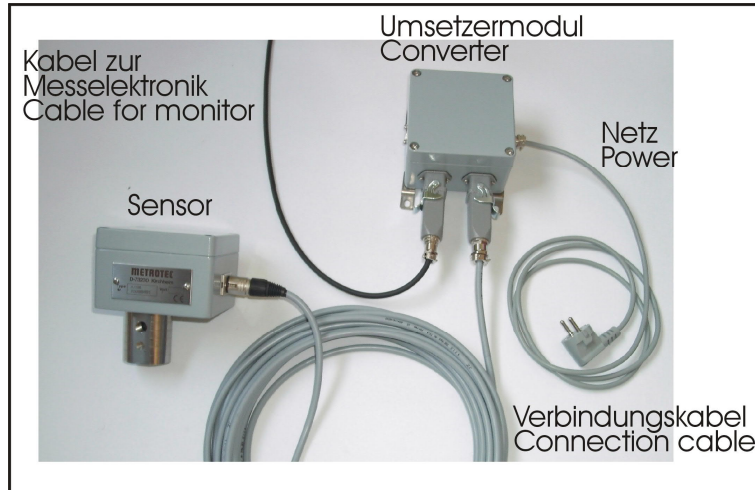
Verschaltung des Sensors A15-N mit dem Umsetzermodule Z15
